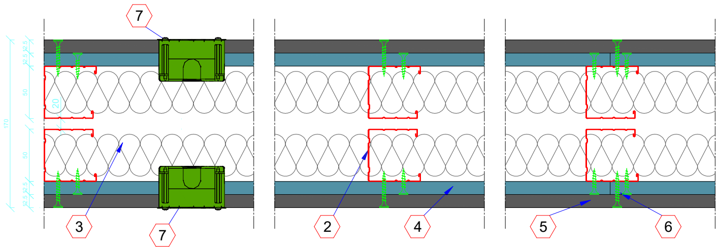
Particolare della sezione A-A Section A-A detail
