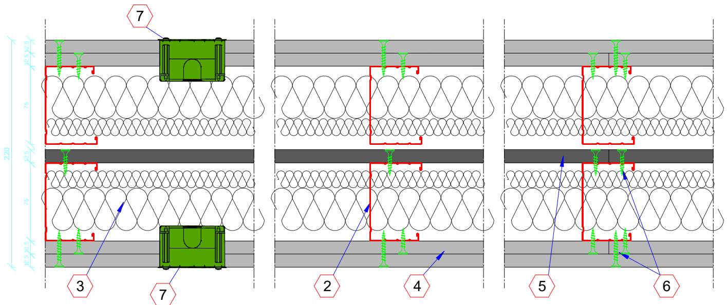
Particolare della sezione A-A
