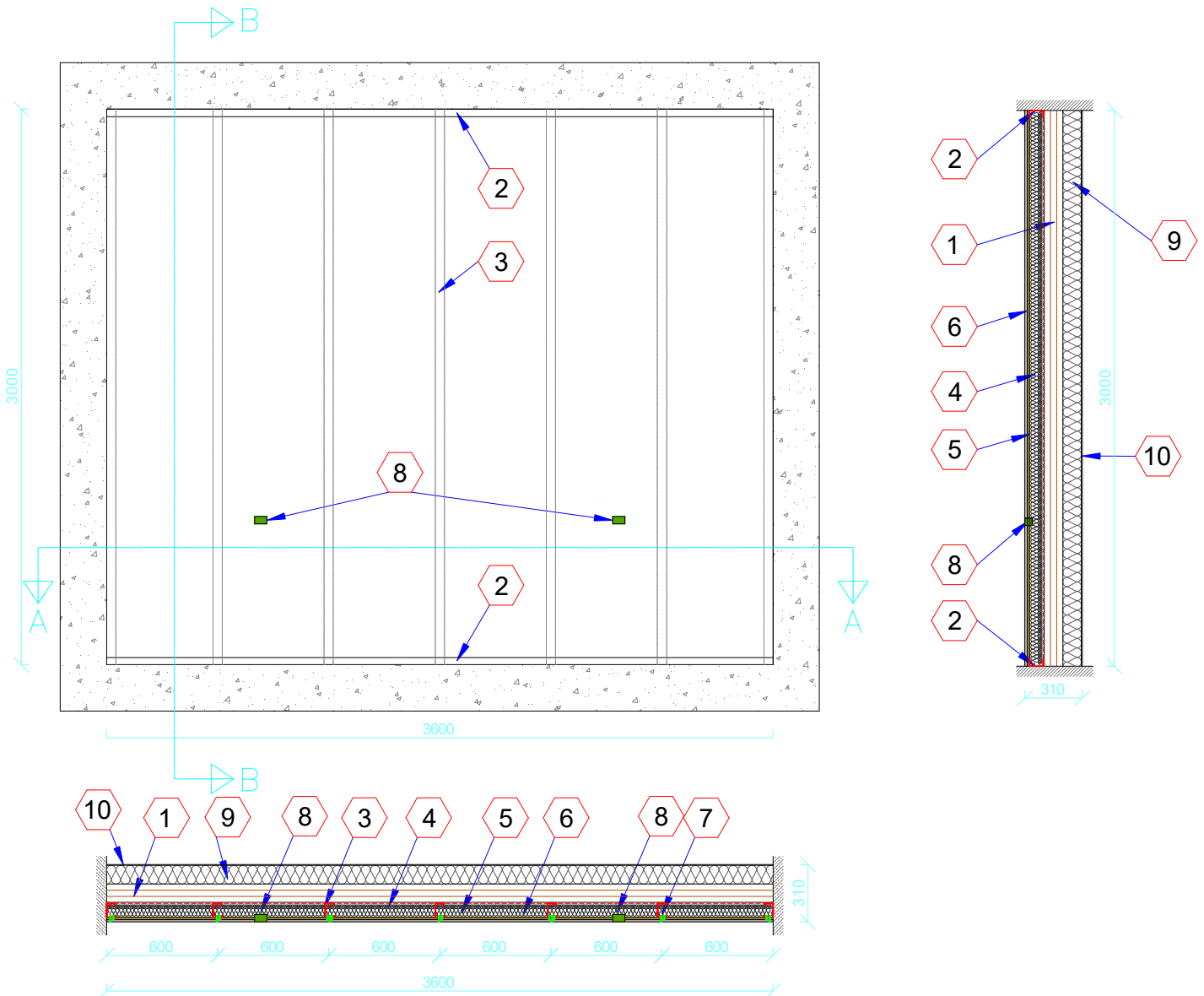
Prospetto e sezioni Elevation and sections
